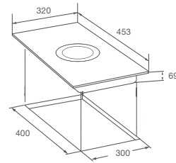
HOB D7RW EIG30102
