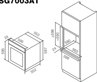
OVEN KSG7007A KSG7003AT
