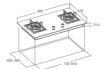
HOB GEG88201 GEG88306-i GHG88215
