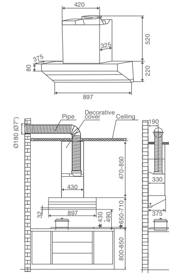
HOOD ZMG9056 / ZMG9057
